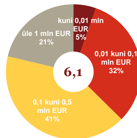
Joonis 7. vDRG jagunemine rahalises vääringus, 2014
