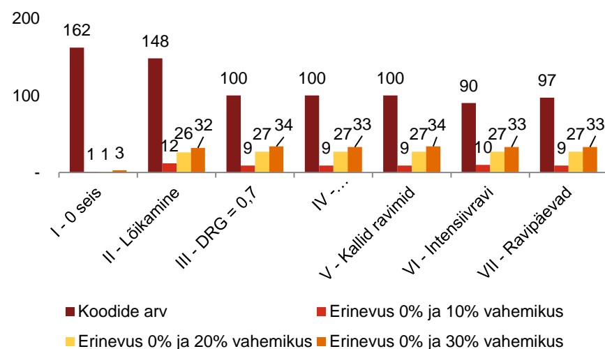
Joonis 15. vDRG empiiriliste ja teoreetiliste piiride suhteline erinevus
