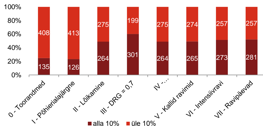
Joonis 31. Test 1: mediaani ja keskväärtuse suhteline erinevus
