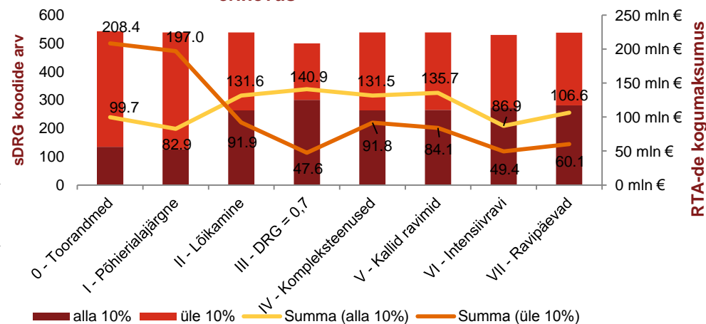
Joonis 32. Test 1: mediaani ja keskväärtuse suhteline erinevus
