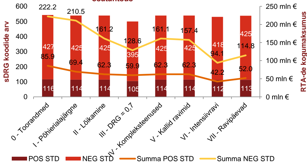
Joonis 30. Negatiivse alumise STD piiriga sDRG koodide osatähtsus
