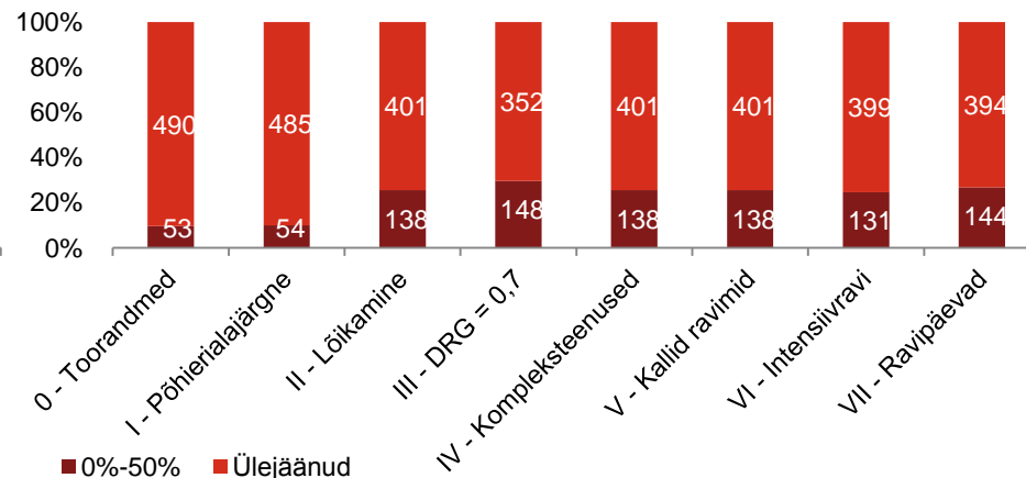
Joonis 39. Test 2: empiiriliste ja teoreetiliste piiride suhteline erinevus 0%-50%
