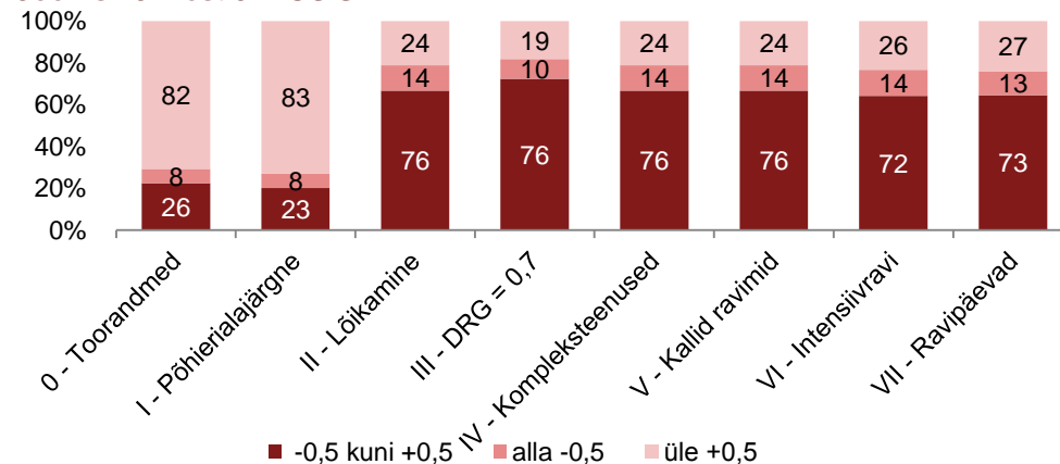
Joonis 49. Test 3: POS STD
